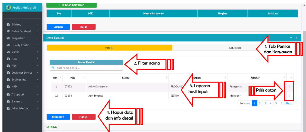
Gambar 4. Halaman Laporan
